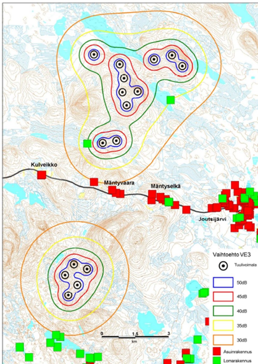
Kuva 8. Kangaslamminvaaran ja Untamovaaran VE3 melumalli sekä lähimmät asuin- ja lomarakennukset
